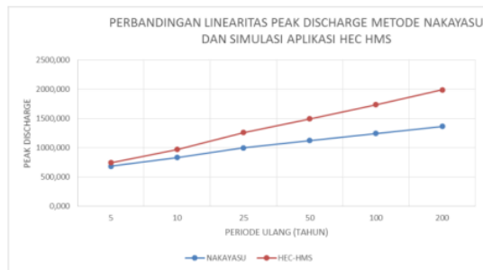
Grafik 3 . Grafik Linearitas Peak Discharge Metode Nakayasu dan HEC-HMS
