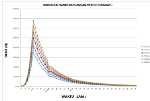
Gambar 1 : Grafik Rekapitulasi Hidrograf Nakayasu
